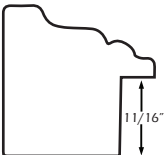
AP-208 1-9/16" x 1-9/16"
