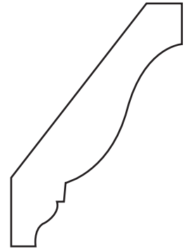
AP-543 7/8" x 4-3/8"
